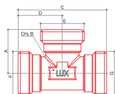
RT 911 Raccordo a T.
